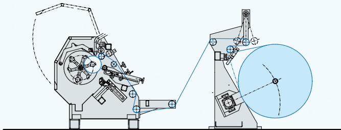
MPW mit Wendestern und drei Wickelwellen
